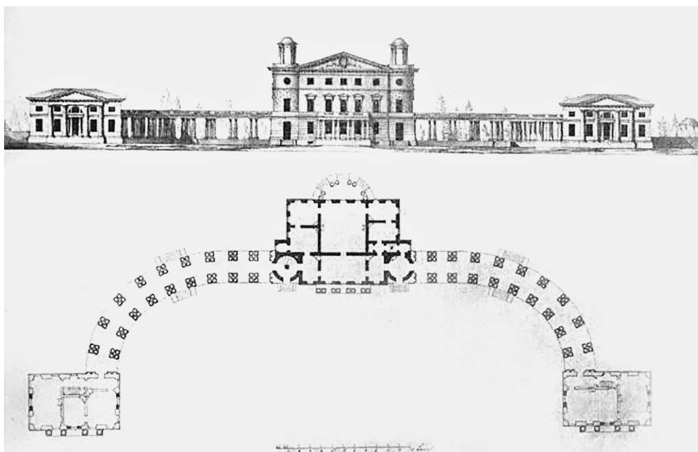
Рис. 30. Рисунок и план первого этажа дачи графа Кушелева-Безбородко [38]
