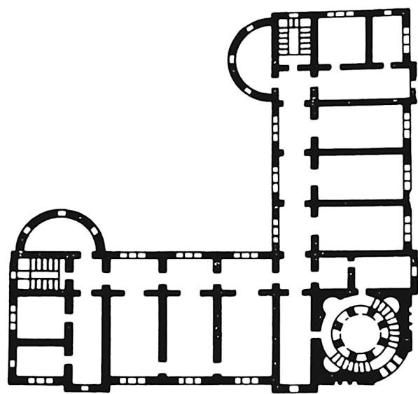
Рис. 21. Женское отделение Обуховской больницы. План второго этажа [27]
